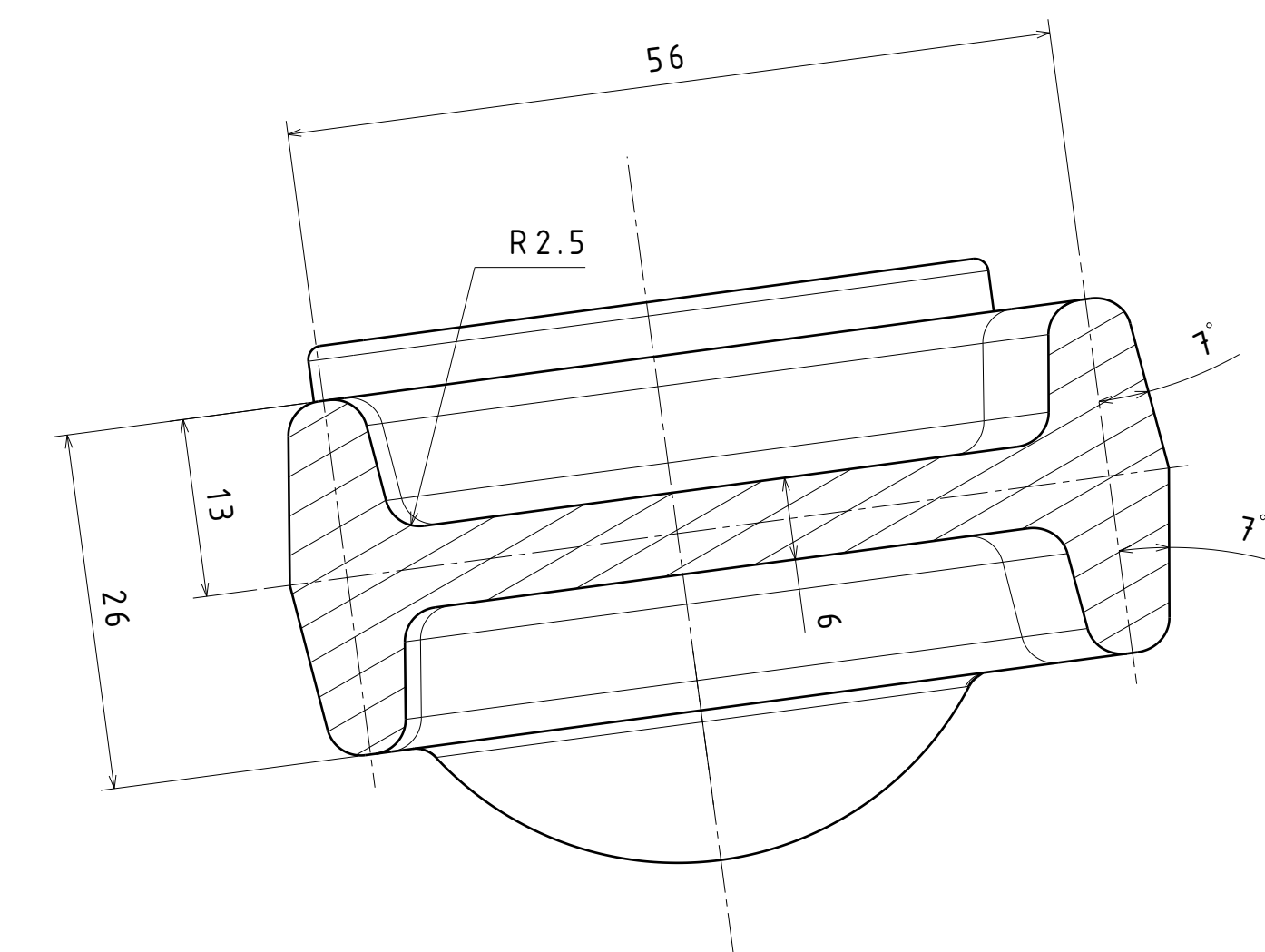
D-D (2:1)
