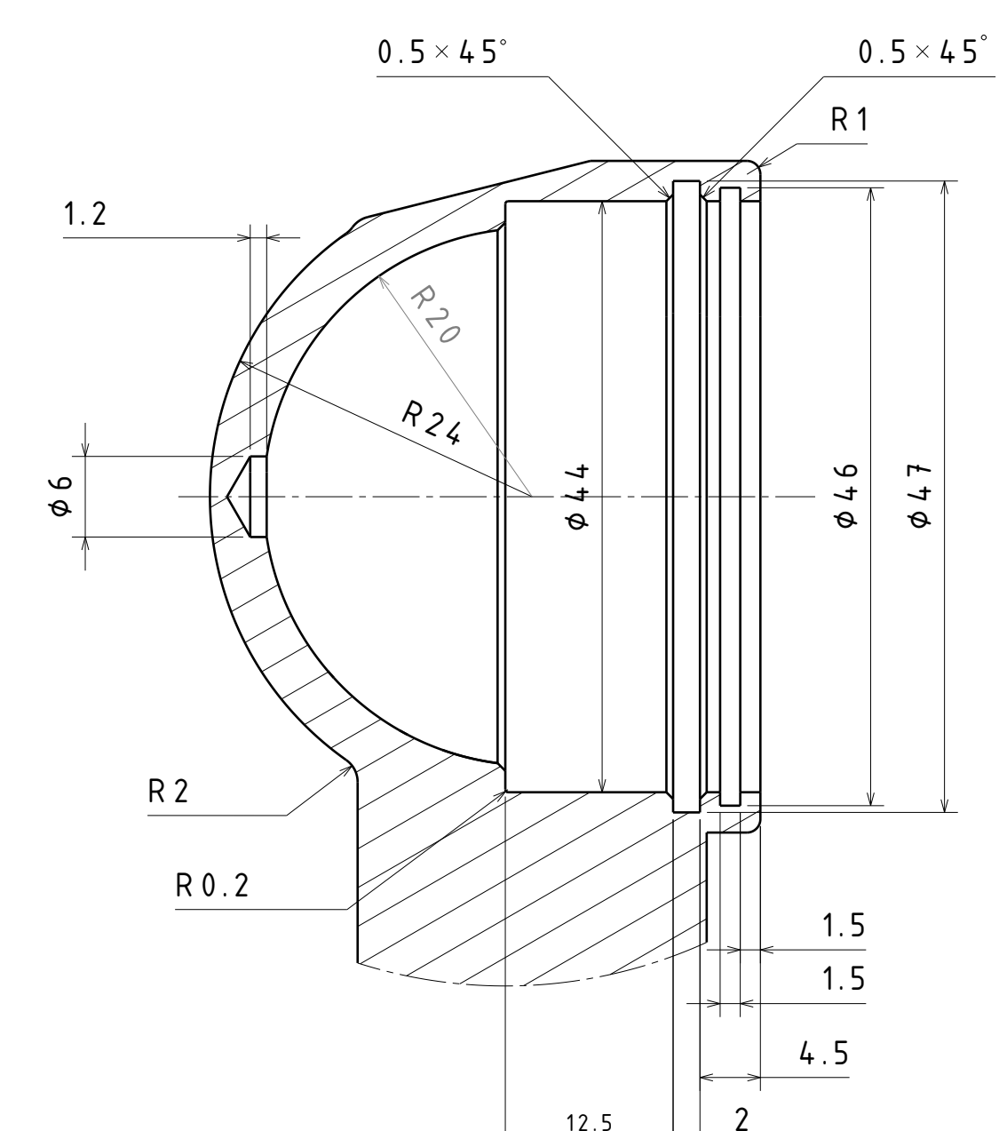
E (2:1)
